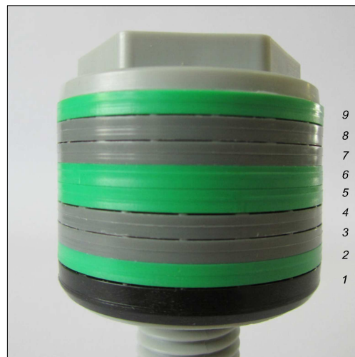
esempio D4.9 - 4 dischi ciechi example D4.9 - 4 blanked disks
